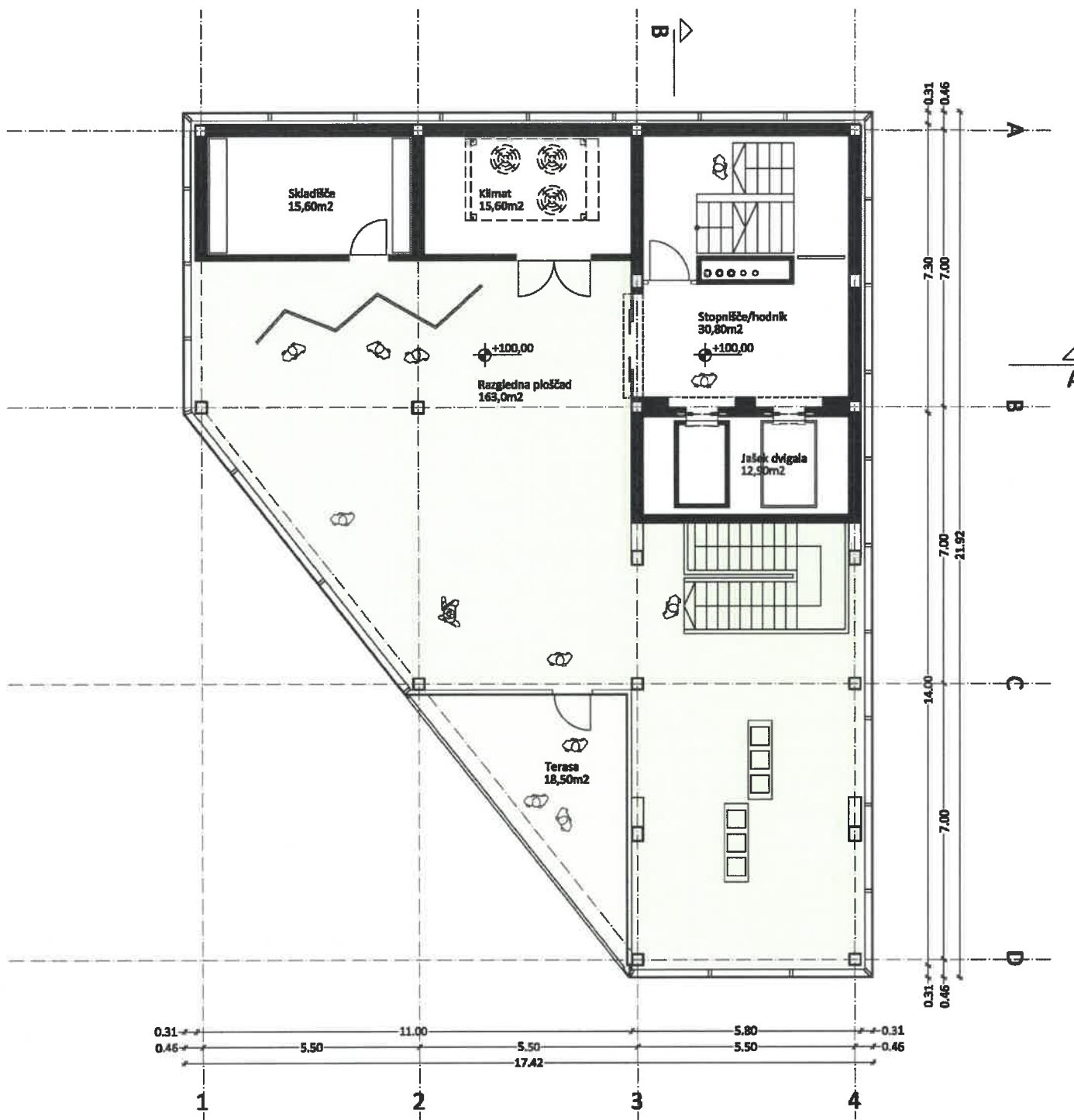
Tloris 2. Etaže M 1:100
