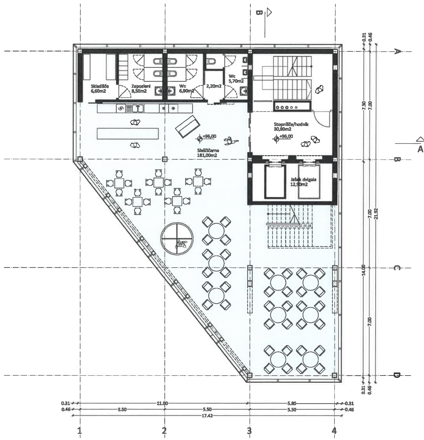
Tloris 1. Etaže M 1:100
