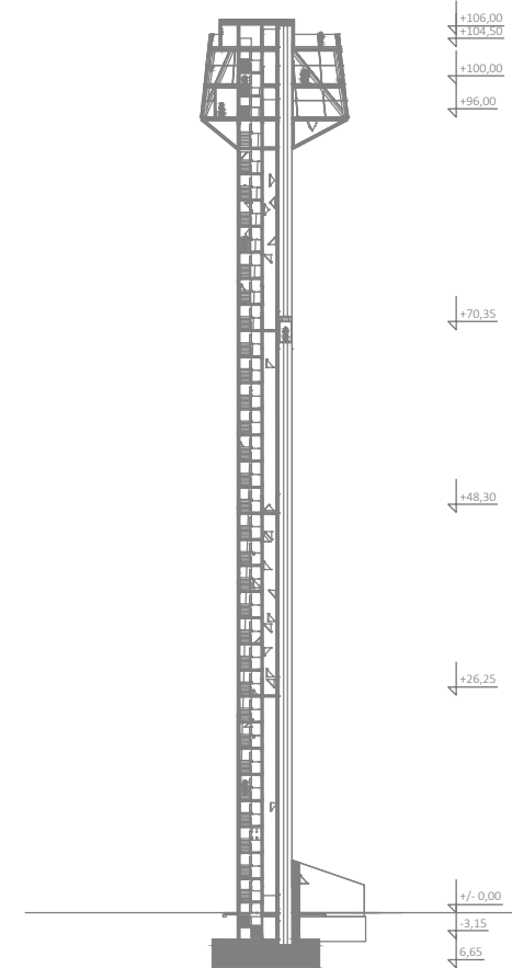
SHEMATSKI PREREZ C - C
