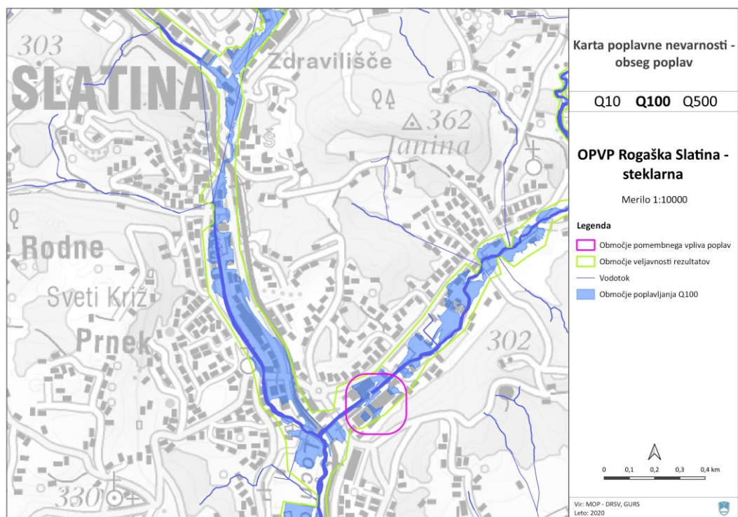
Slika 4: Karta poplavne nevarnosti - obseg poplav Q100
