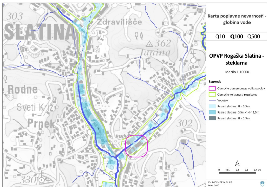
Slika 6: Karta poplavne nevarnosti - globina vode Q100
